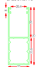
GU7527 CASSONETTO
